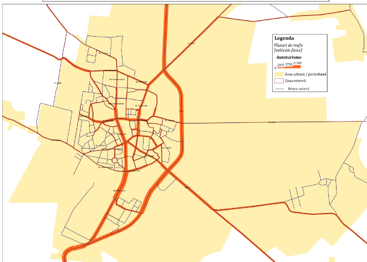
Figura 3.48. Fluxuri de trafic, autoturisme, MZA 2015.
