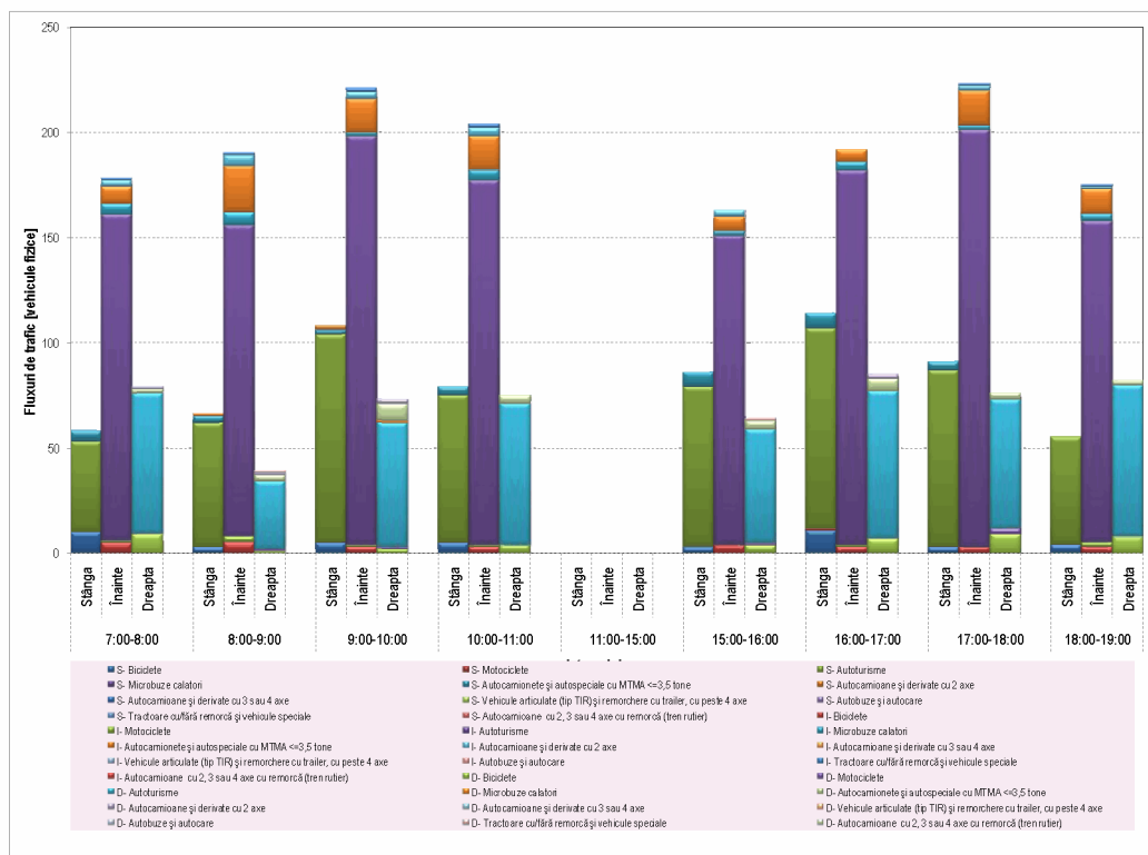
Figura 3.29. Distribuția orară a volumelor de trafic. Postul 10, Brat - Str. Unirea Principatelor.
