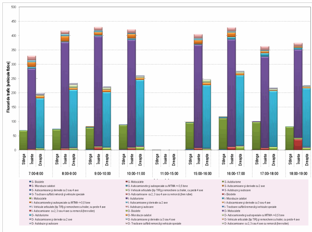
Figura 3.28. Distribuția orară a volumelor de trafic. Postul 10, Brat - Bdul Unirii Sud.
