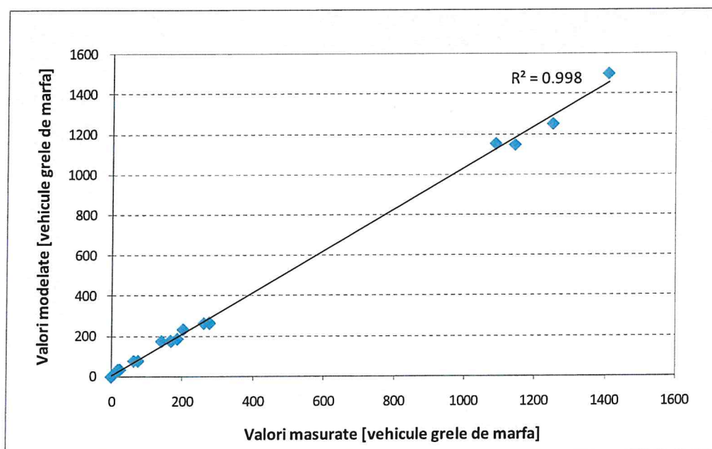
Figura 3.60. Rezultatele analizei afectării, autovehicule grele de marfă.
