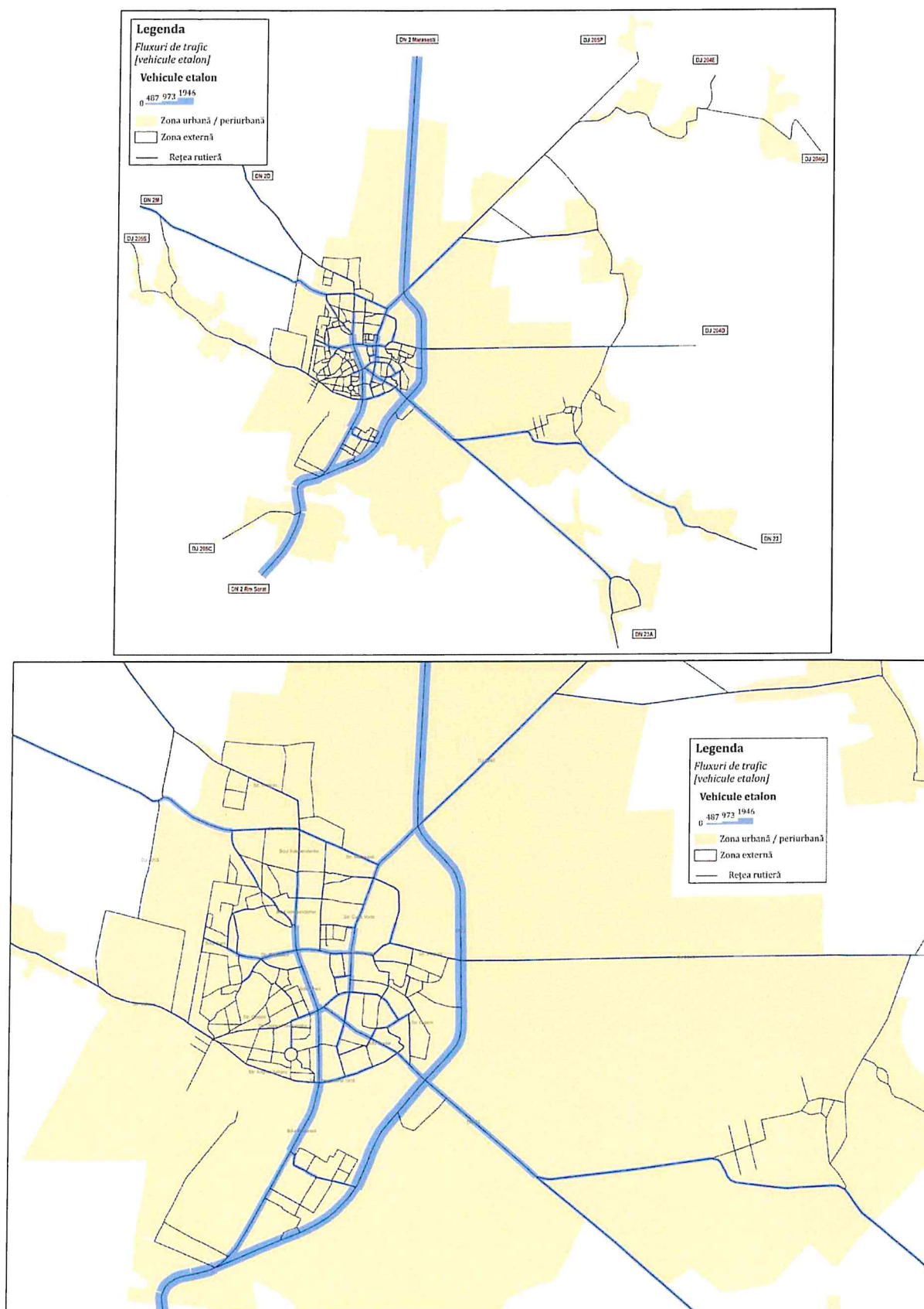
Figura 3.55. Fluxuri de trafic, vehicule etalon, ora de varf de trafic, 2015.
