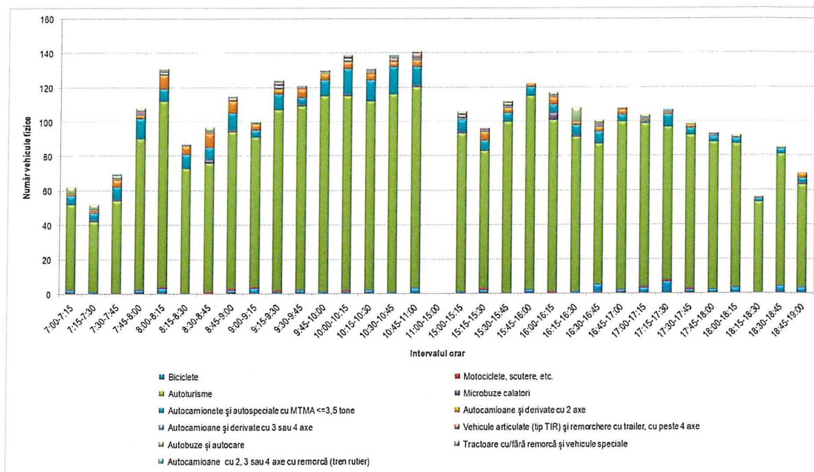
Figura 3.25. Distribuția orară a volumelor de trafic. Postul 7.
