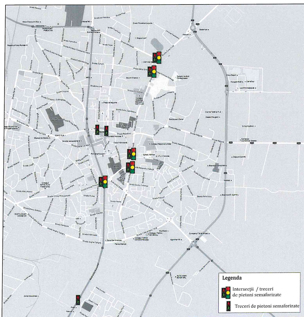
Figura 2.44. Sistemele de semaforizare actuale.
