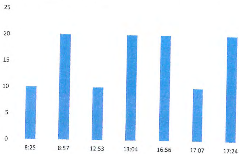
Fig. 2.96. Linia 1 - evoluția gradului de umplere a vehiculelor de-a lungul intervalelor de timp monitorizate
