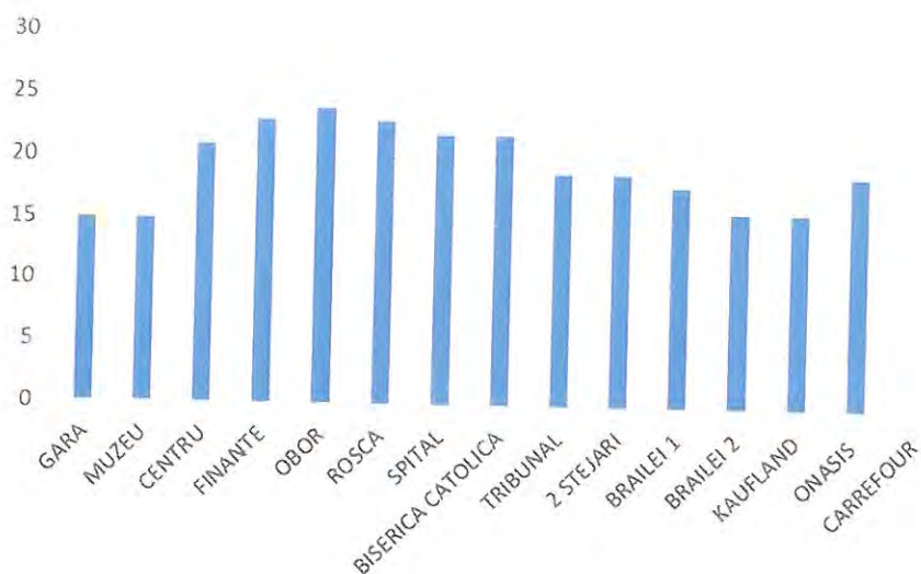
Fig. 2.66. Linia 7 - evoluția gradului de încărcare de-a lungul traseului, interval prânz, tur
