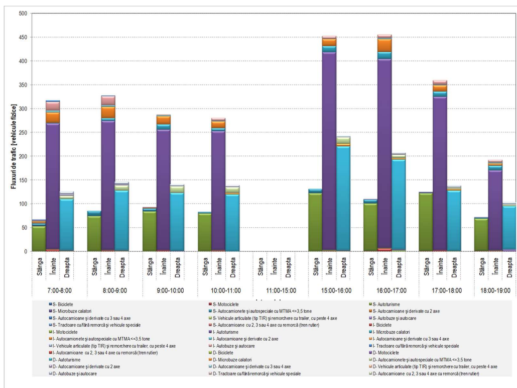
Figura 3.37. Distribuția orară a volumelor de trafic. Postul 12, Brașov - Str. Cuza Vodă Nord.
