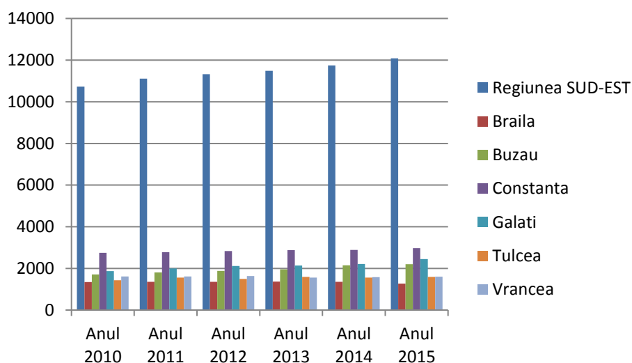
Fig. 7.17. Lungimea totală simplă a rețelei de distribuție a apei potabile în perioada 2010-2015
