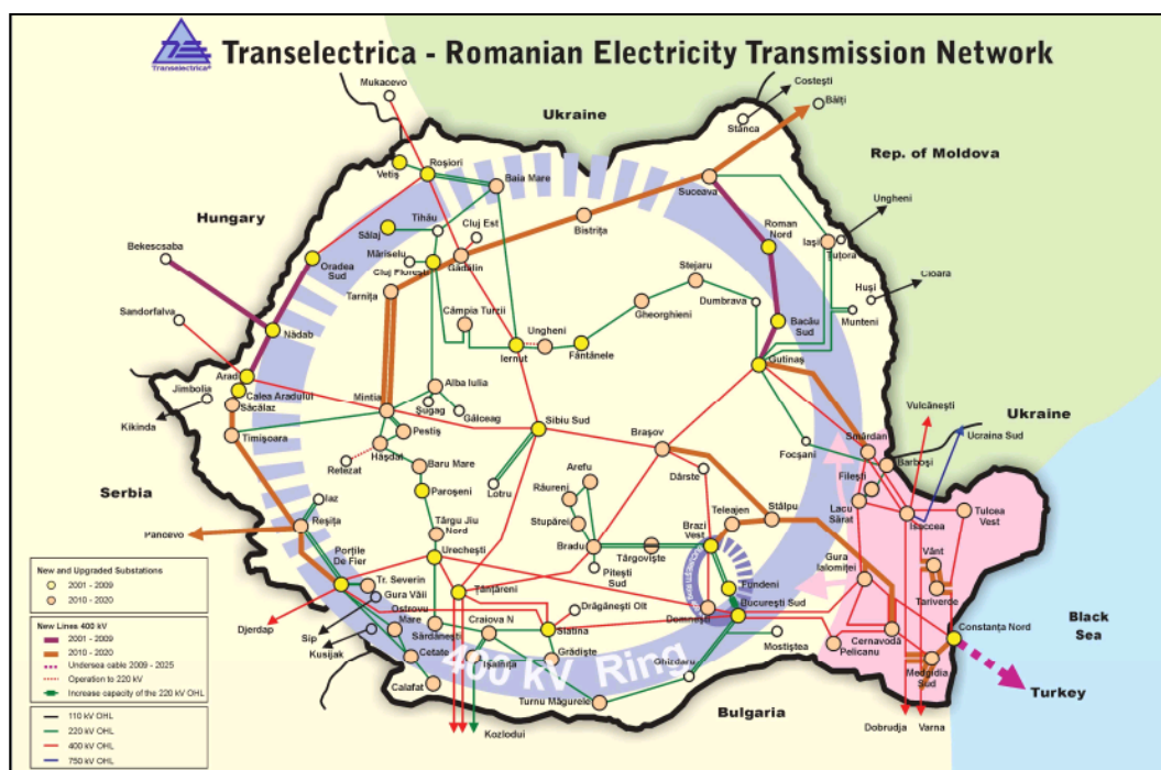
Fig. 7.28. Rețeaua națională de transport a energiei electrice 173
