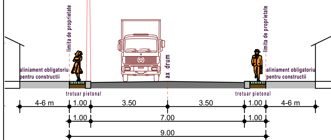
PROFIL 1 - 1 9.00 m
