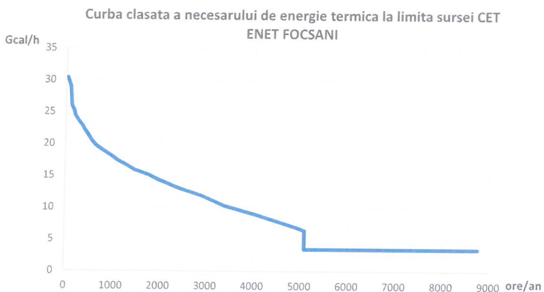
Figura 6-6: Curba clasată a necesarului de energie termică la limita sursei CET ENET
